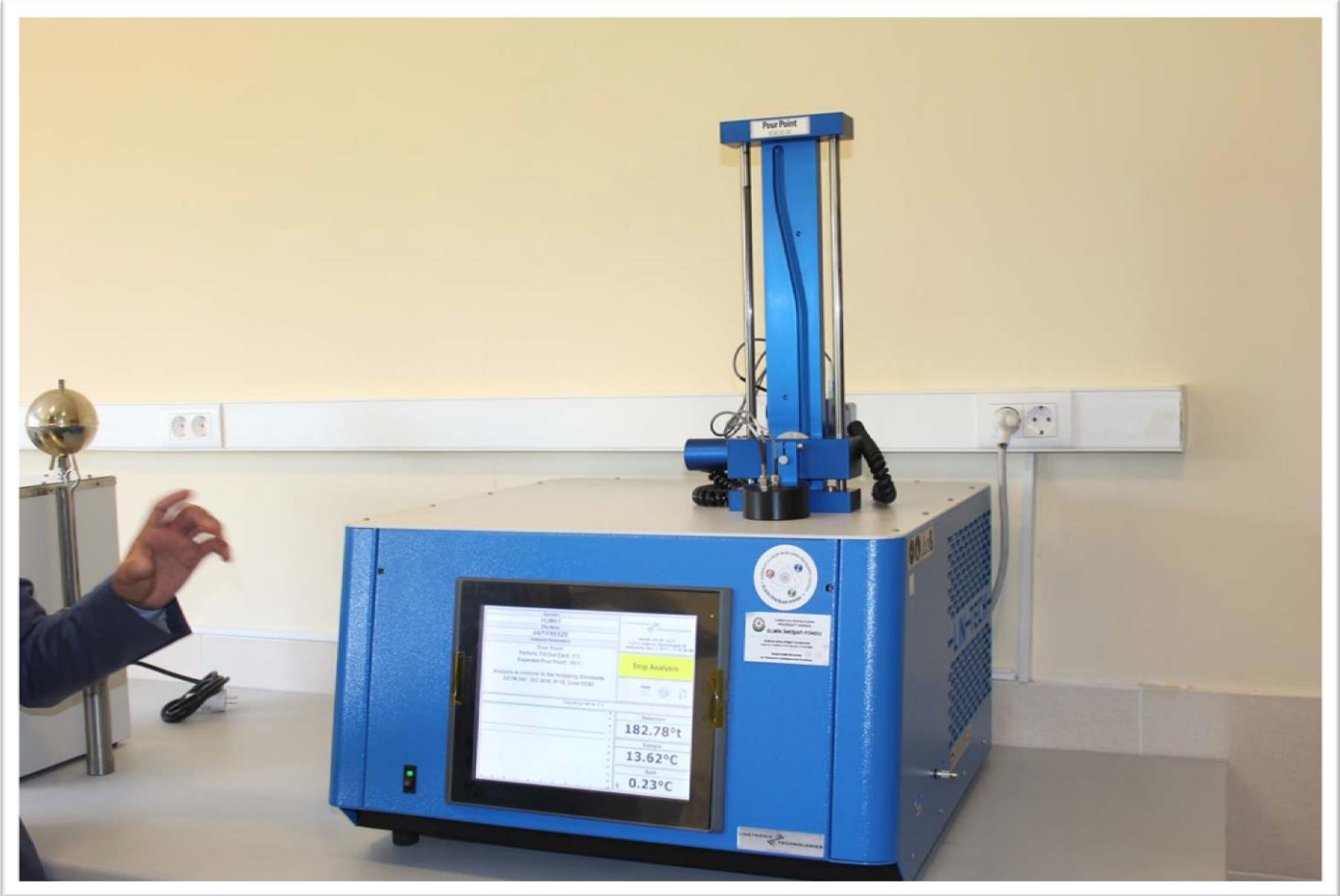
POUR POINT NEW LAB 300/2. Donma temperaturunu təyin edən cihaz, İSO 2160 ASTM D 97 üzrə.
