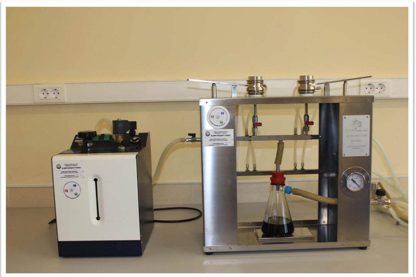
TOTAL SEDIMENT 1150. Yağlarda mexaniki qarışıqları təyin edən cihaz, ASTM D473 üzrə.
