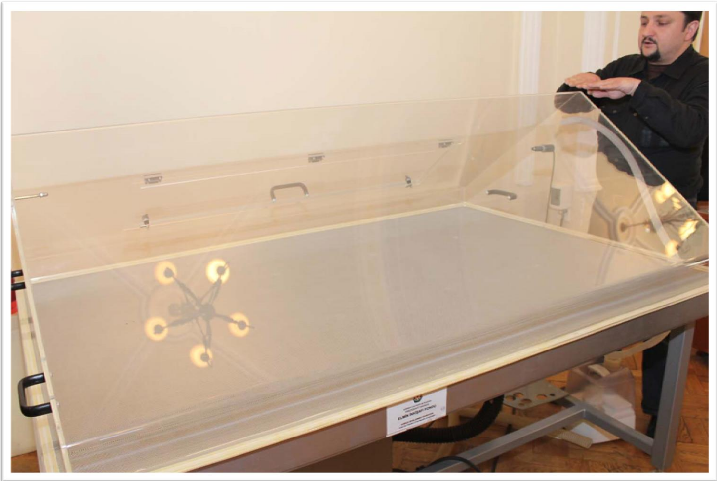
Balkon təmizləmə masası. Masa arxeoloji tekstil və kağız üzərində olan tarixi sənədləri və qrafik əsərləri bərpa etməyə geniş imkanlar yaradır.
